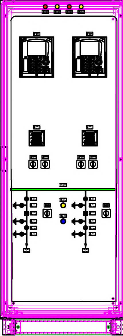
п.6 Защита, управление и автоматика 35ВЛ Сукля- IIп. | 35ВЛ Сукля- Iп.
