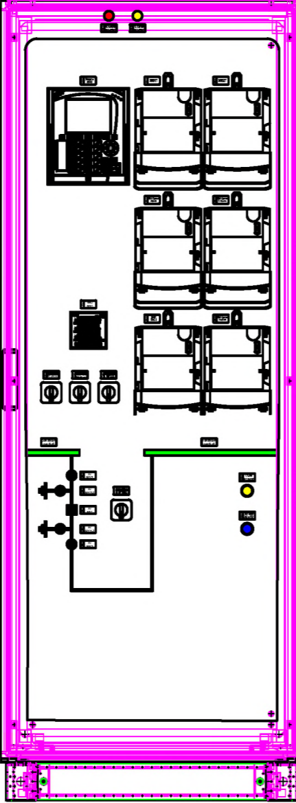
п.7 Защита, управ. и автоматика 35ВС Учет стороны 35 кВ (ВВ,ВЛ)
