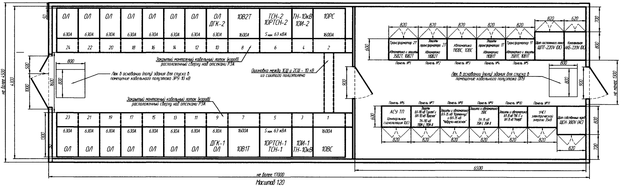
Приложение №1: План размещения электротехнического оборудования в блочно-модульном здании ОПУ и ЗРУ-10кВ на п/ст "Слободзья 110/35/10 кВ"
